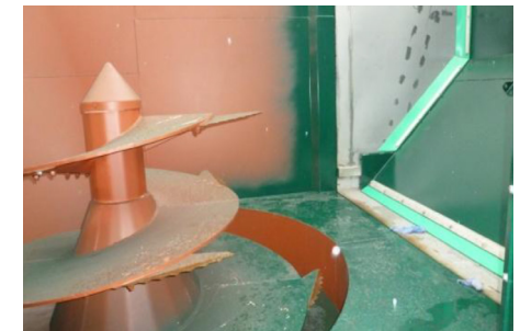
angekoppelter Mischer mit 400 mm Abbruchkante
