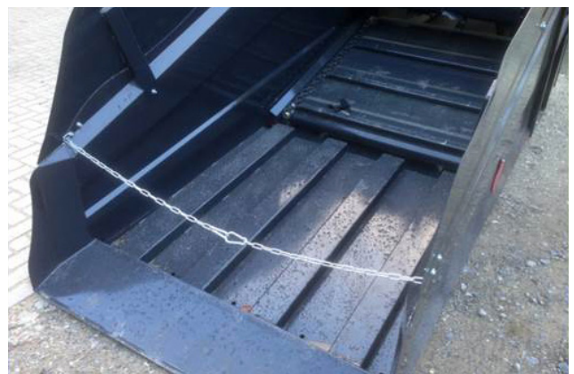
optional Kastenverlängerung für Heu und Stroh
