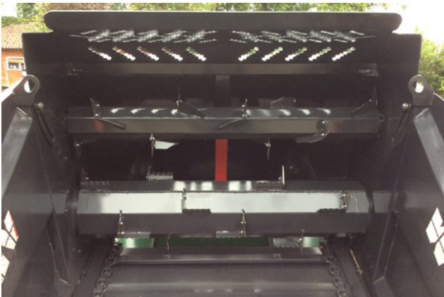
2 hydr. angetriebene Auflösewalzen
