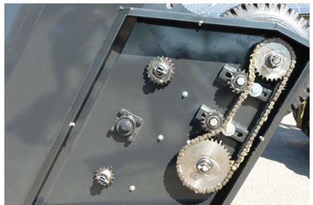
Geschwindigkeits- und Mengendosierung über Wechselkettenräder
