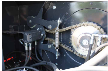
elektrohydraulischer Antrieb mit intelligenter Steuerung
